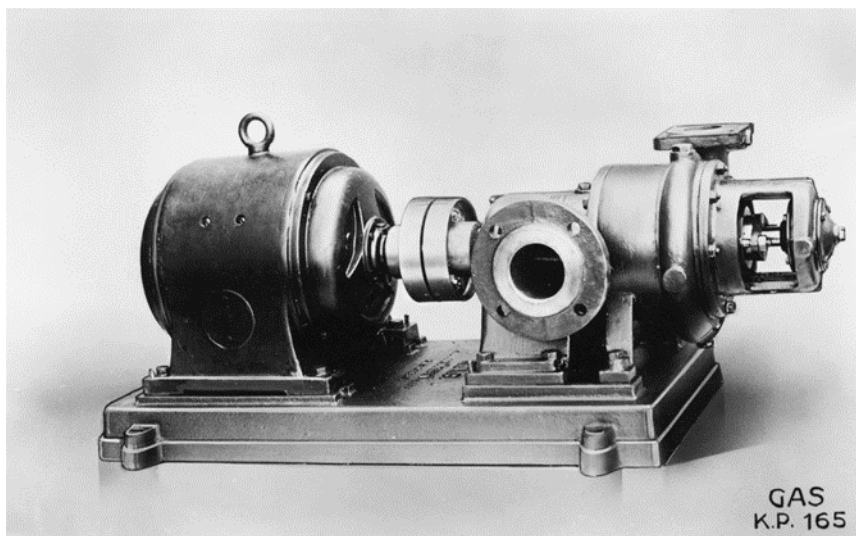
Insinööri Emil Oeschin suunnittelema ensimmäinen mänttäläinen teollisuusprosessipumppu, tyyppi D
